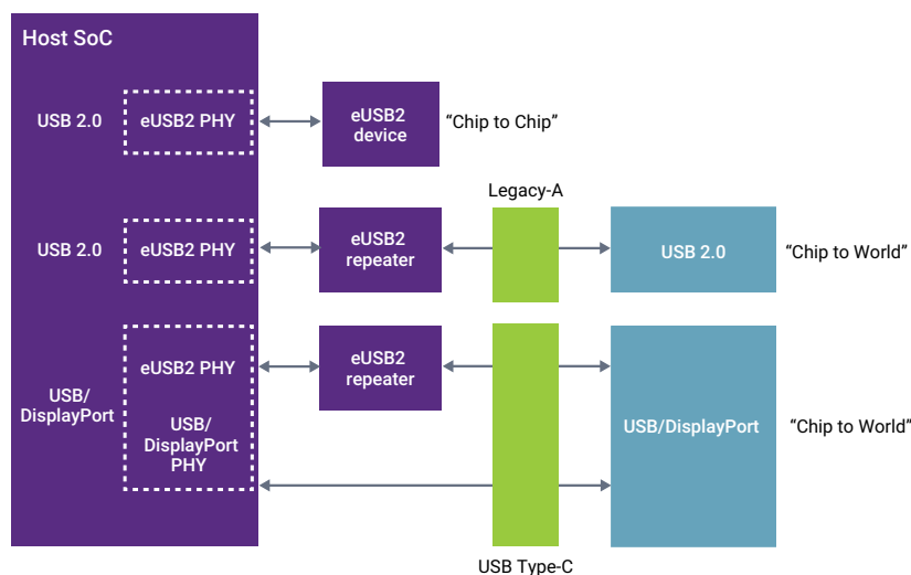
图1:eUSB2用例
