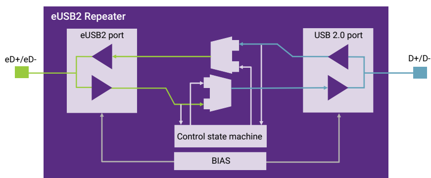
图3:eUSB2中继器框图
