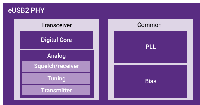
图2:eUSB2 PHY框图
